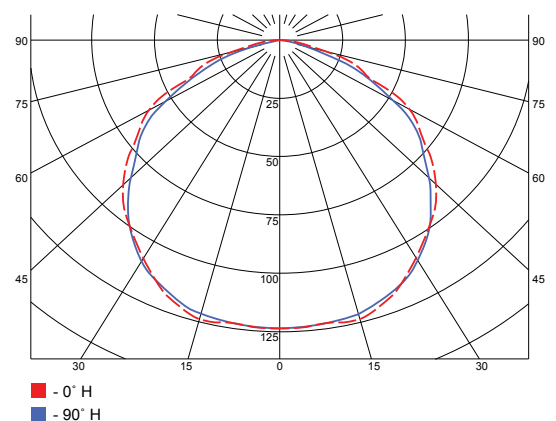
Lichtverteilungskurve
